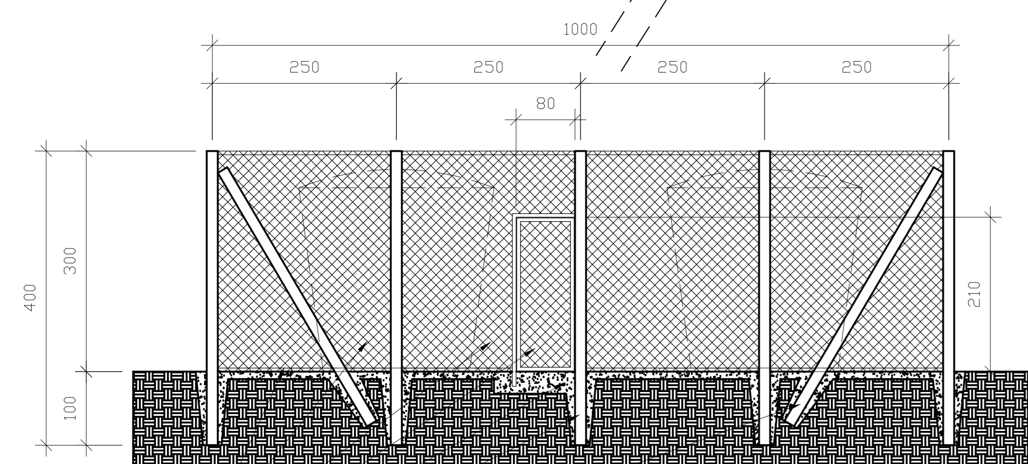
3 ESQUEMA CISTERNA ESCALA 1:50
