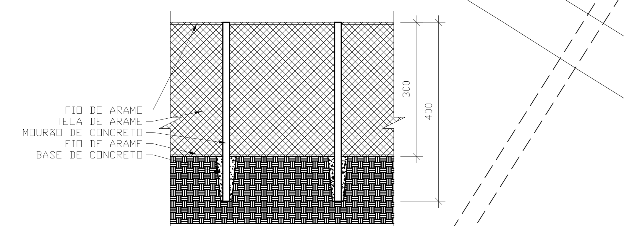
2 ESQUEMA CERCA VIVA ESCALA 1:50
