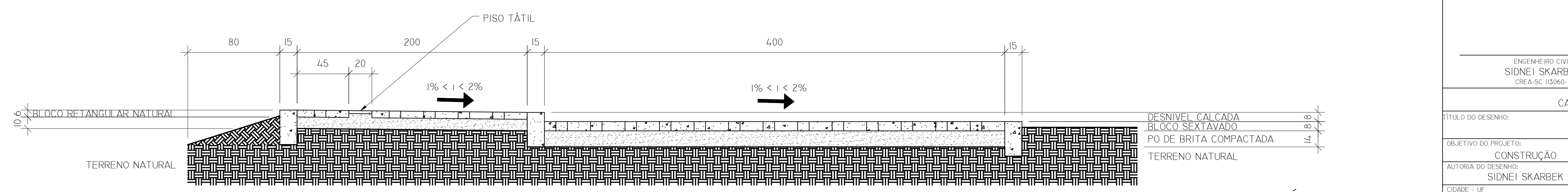
CORTE ESQUEMÁTICO VIAS 4M ESC: 1/20
